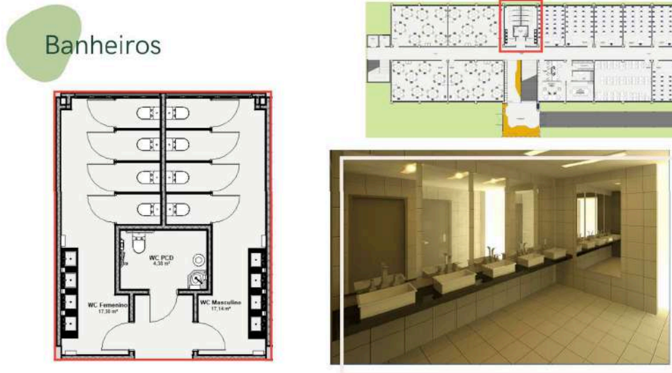
Figura 04 – Banheiros acessíveis
